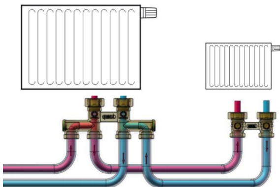
Radiatorinkoppling vid högeranslutning;
