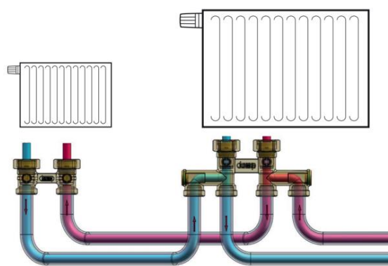
Radiatorinkoppling vid vänsteranslutning;
